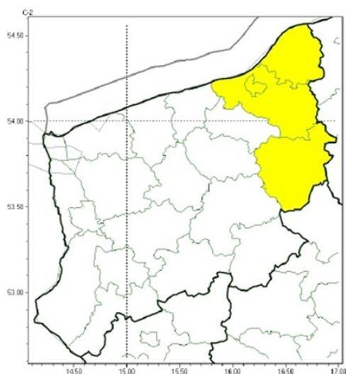
Oblodzenie
