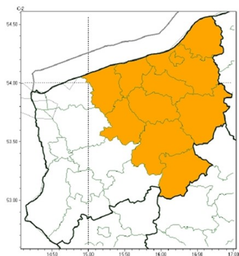
Opady marznące
