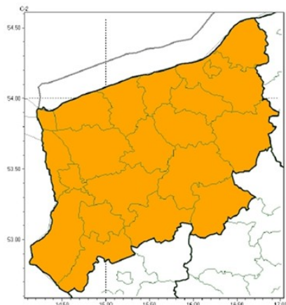
Opady marznące
